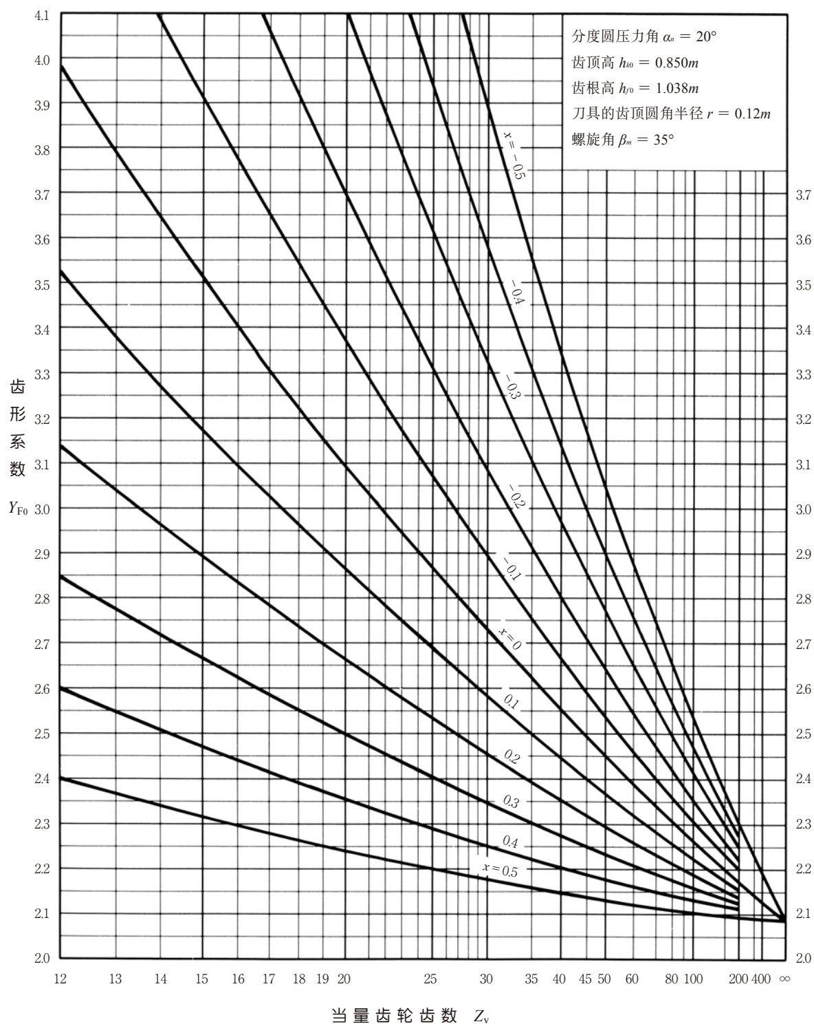
图 10.9 齿形系数 Y_{F0} (弧齿锥齿轮)
