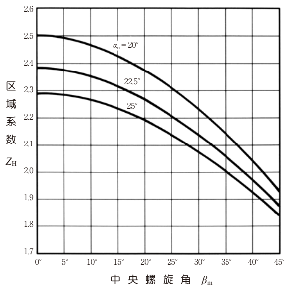
图 10.10 区域系数 Z_H
