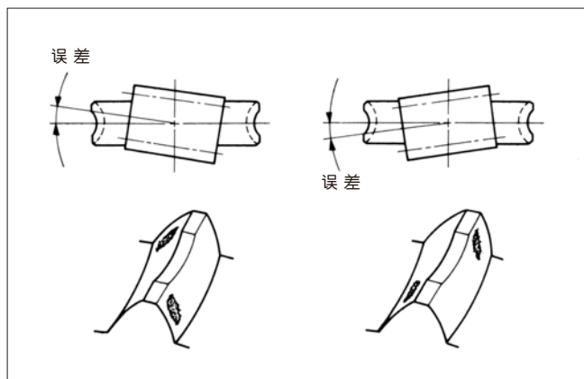
图 8.7 齿轮箱有轴角误差时的轮齿接触
