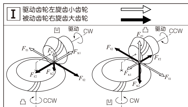
图 12.5 弧齿锥齿轮的旋转方向与轮齿的受力
