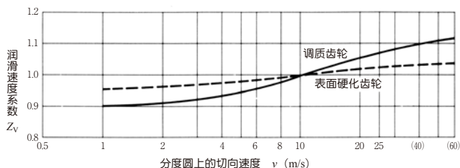
图 10.5 润滑速度系数 Z_V
