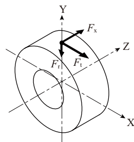
图 12.1 轮齿的受力示意图
