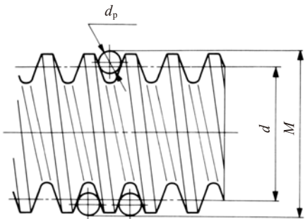
图 5.10 蜗杆的三量柱法
