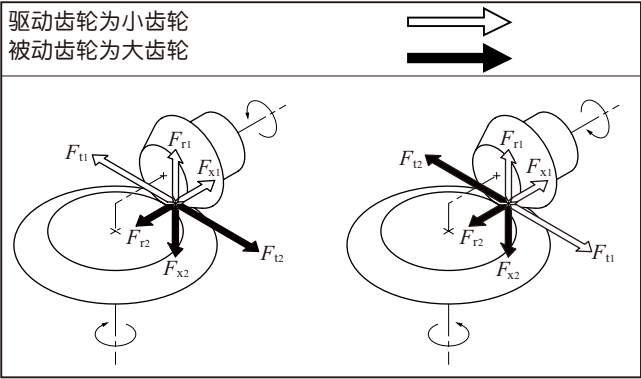
图 12.3 直齿锥齿轮的旋转方向与轮齿受力
