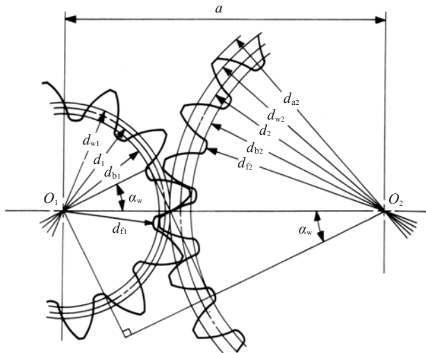
图 4.2 变位齿轮的啮合
