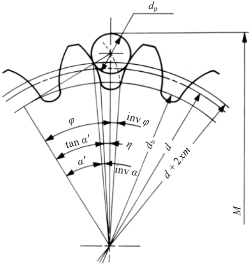
图 5.7 正齿轮的量柱跨距
