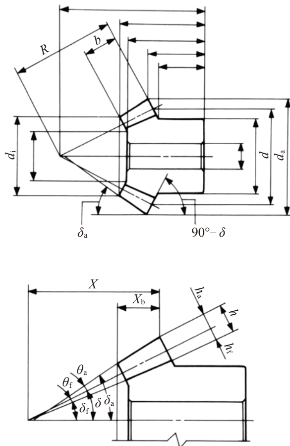
图 4.10 锥齿轮的尺寸及角度
