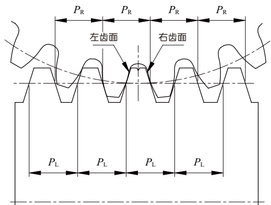
图 6.7 双导程蜗杆副原理图
