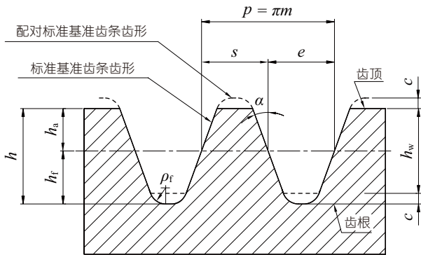
图 3.1 基准齿条齿形
