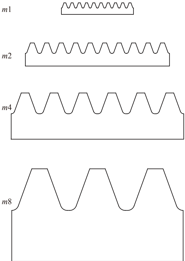
图 3.2 齿条齿形的模数原寸图
