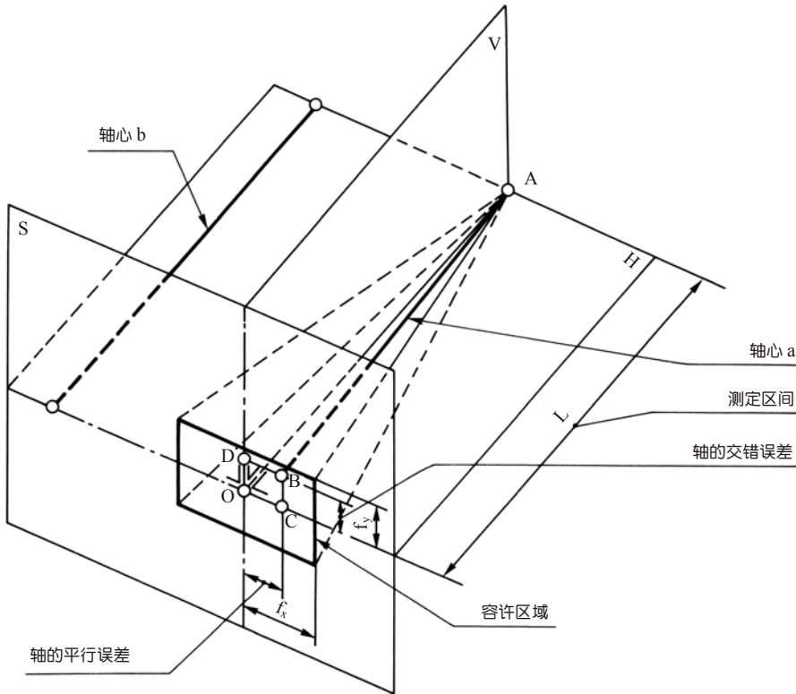
图 8.1 轴平行误差与交错误差
