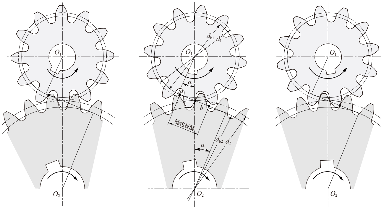
图 3.4 渐开线齿轮的啮合
