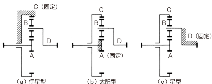
图 17.3 行星齿轮机构的类型
