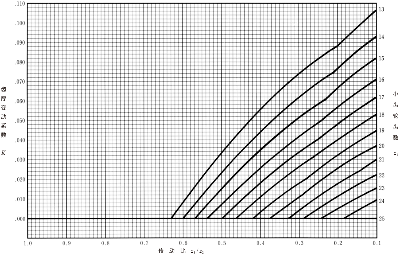
图 5.2 格里森直齿锥齿轮的齿厚变动系数 K 线图
