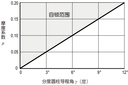
图 4.23 分度圆柱导程角 \gamma 与摩擦系数 \mu 的自锁极限
