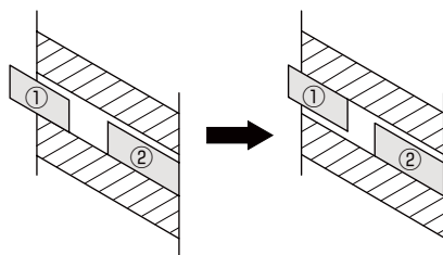
图 6.5 斜齿齿轮的侧隙调整
