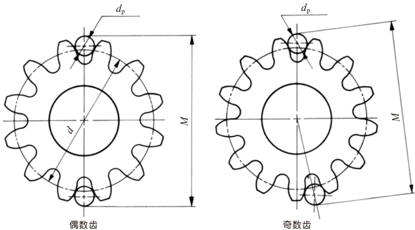
图 5.6 正齿轮的量柱(球)法
