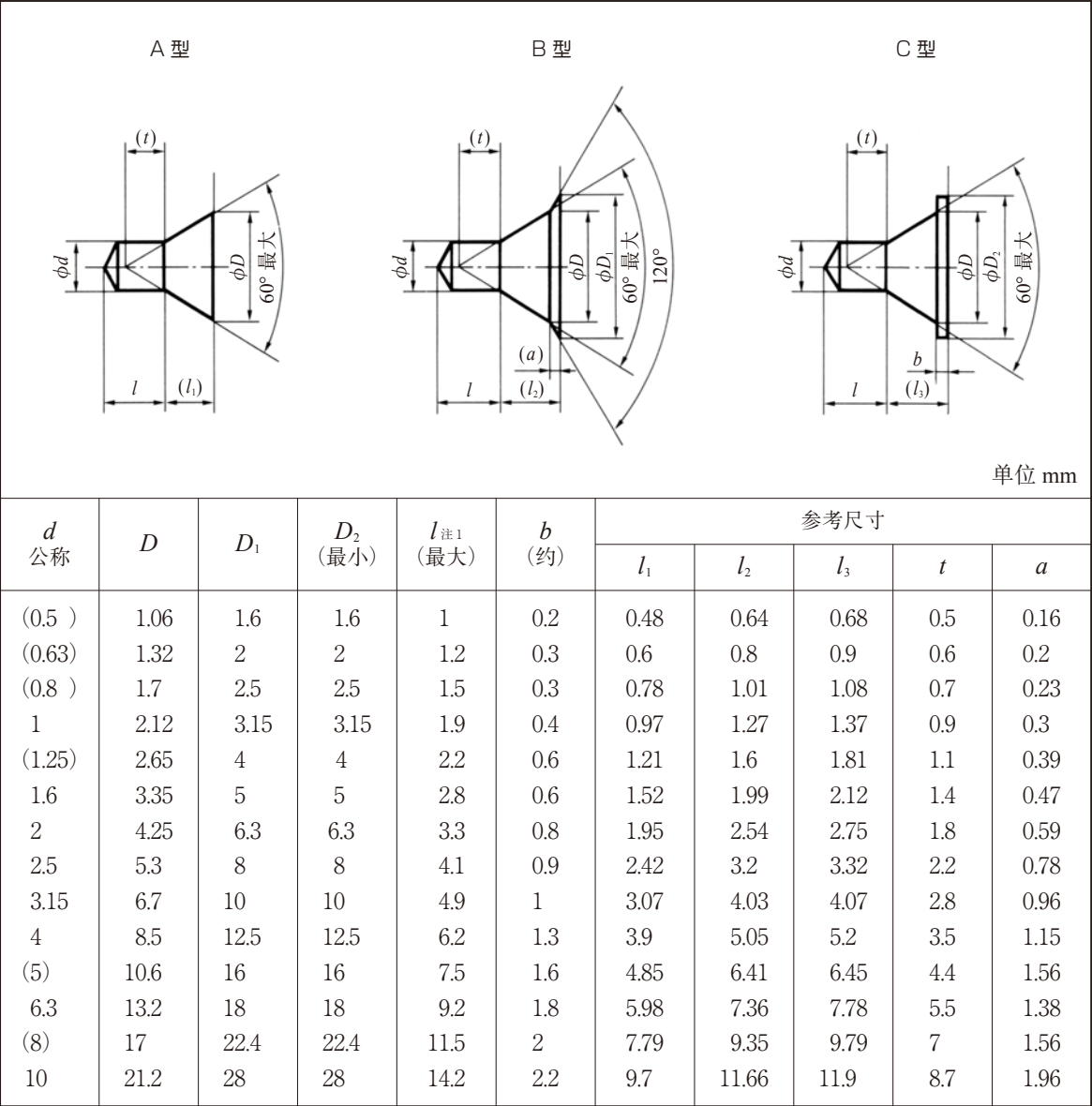
60 度中心孔的形状及尺寸
