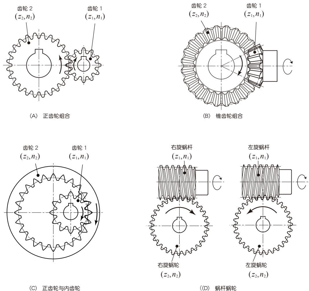
图 2.1 单级齿轮机构
