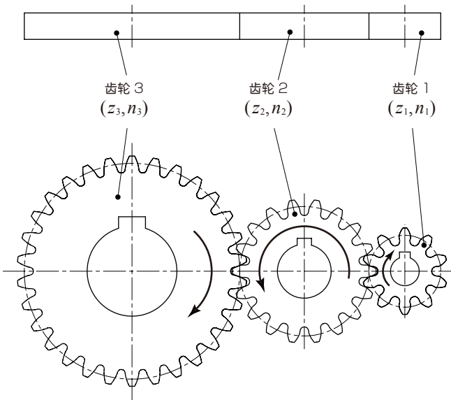
图 2.4 使用了惰轮的单级齿轮机构
