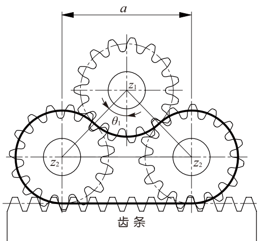
图 17.6 封闭啮合齿轮机构
