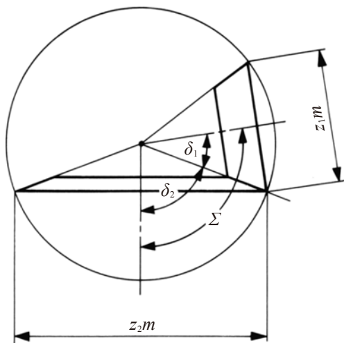
图 4.8 锥齿轮的分度圆锥角
