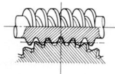
图 1.10 圆柱蜗杆副
