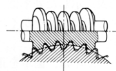
图 1.13 鼓形蜗杆副
