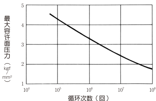
图 11.6 正齿轮的最大面压
