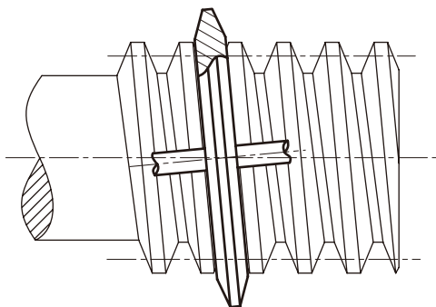
图 4.15 3 形蜗杆的切削及磨削
