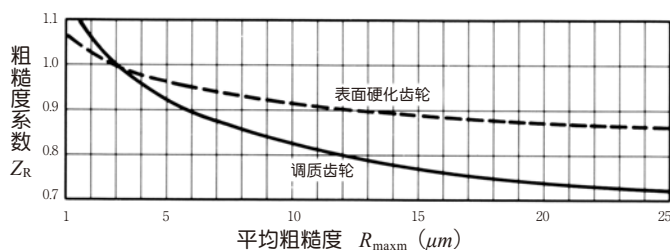
图 10.11 粗糙度系数 Z_R
