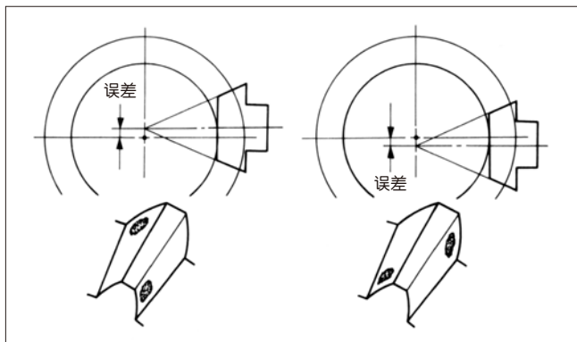
图 8.3 齿轮箱有偏心误差时的轮齿接触
