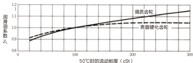
图 10.3 润滑油系数 Z_L
