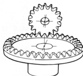
图 1.12 面齿轮
