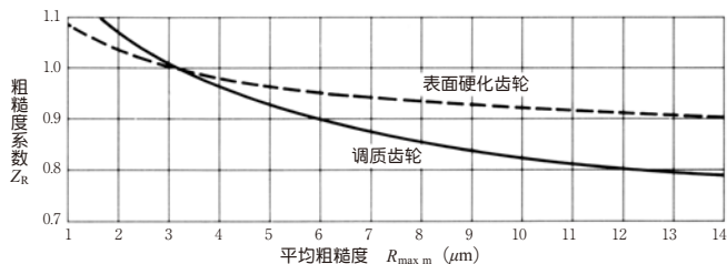
图 10.4 粗糙度系数 Z_R
