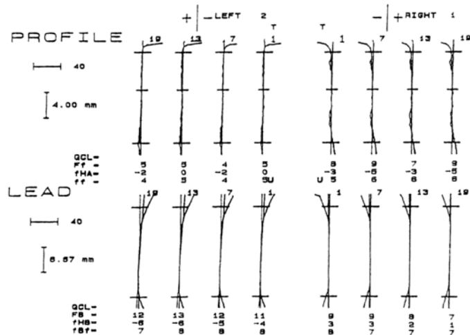
图 7.6 齿形偏差及齿线方向偏差的测定例
