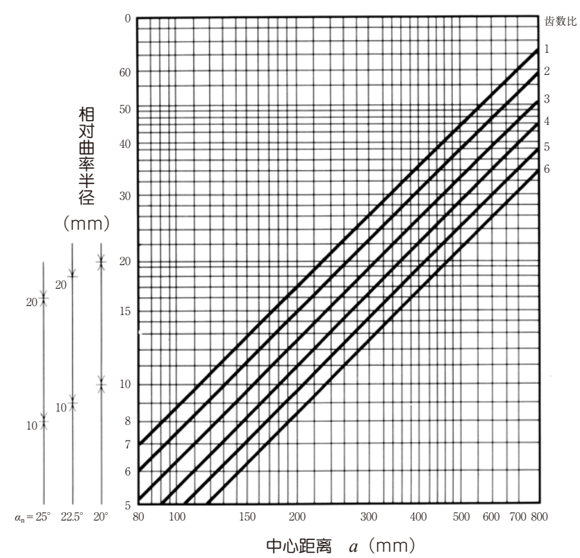
图 10.6 相对曲率半径
