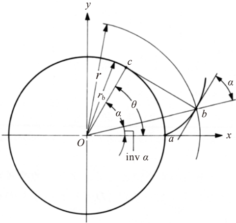
图 3.3 渐开线曲线
