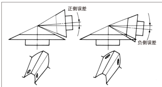
图 8.4 齿轮箱有轴角误差时的轮齿接触
