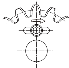
图 6.4 两个重迭齿轮的调节(固定式)
