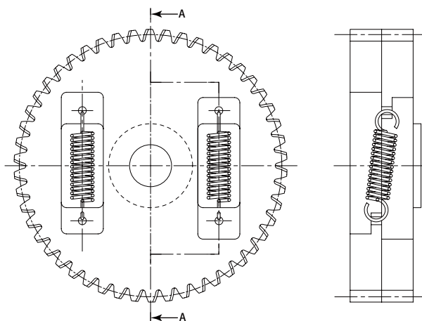
图 6.8 剪形夹齿轮（盘簧使用例）
