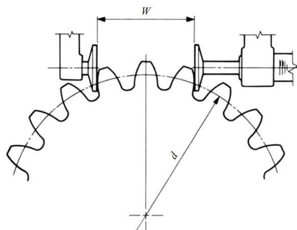
图 5.4 公法线长度法(正齿轮)
