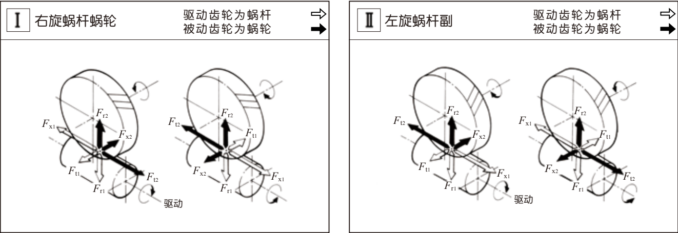
图 12.6 蜗杆蜗轮的旋转方向及轮齿受力
