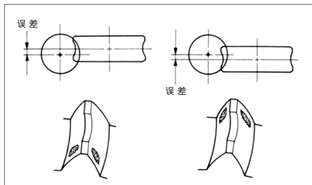
图 8.9 蜗轮有安装位置误差时的轮齿接
