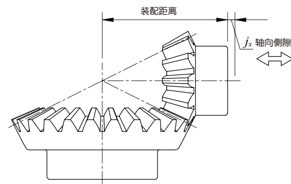
图 6.2 锥齿轮的轴向侧隙
