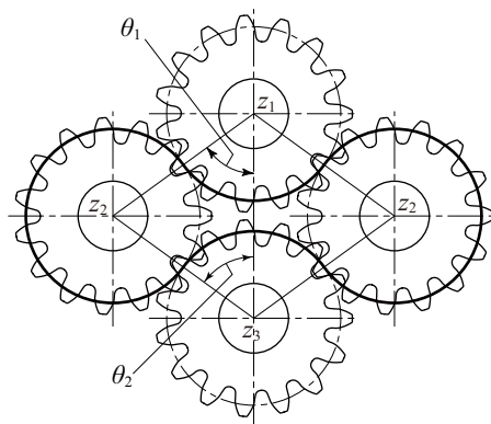
图 17.5 封闭啮合齿轮机构
