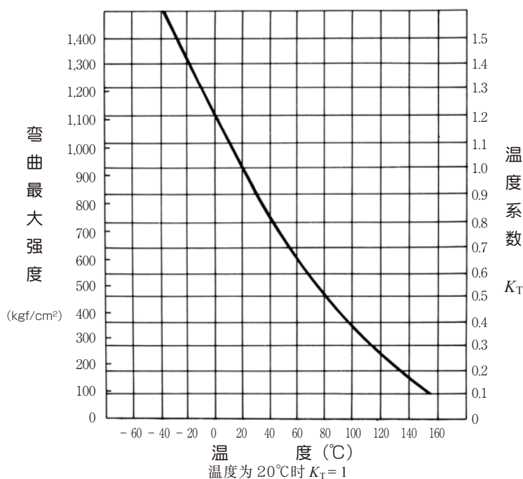
图 11.4 温度系数 K_T
