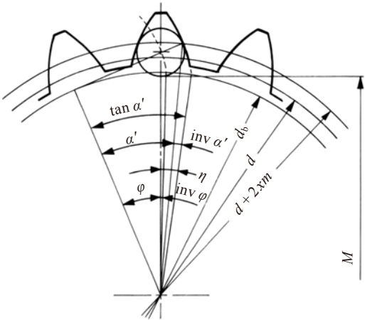
图 5.9 内齿轮的量柱(球)跨距
