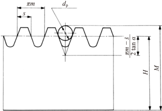
图 5.8 齿条的量柱跨距
