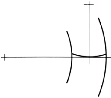
图 4.13 零度锥齿轮 (左旋齿)
