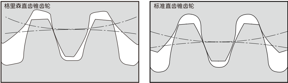
图 4.11 直齿锥齿轮的齿形
