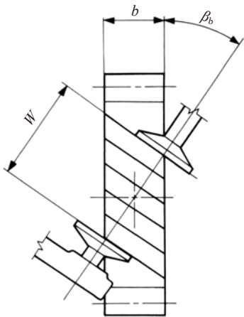
图 5.5 斜齿齿轮的齿宽
