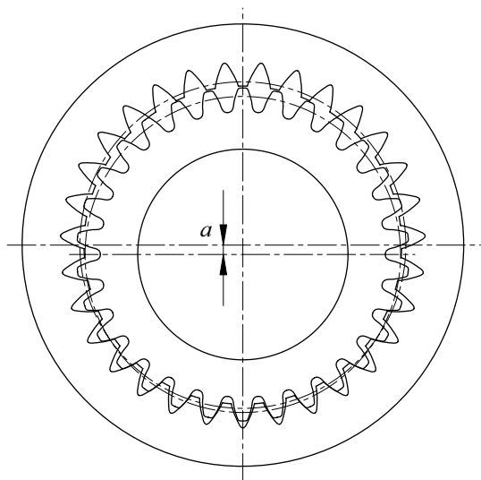
图 17.4 齿数差为 1 的内齿轮与正齿轮的啮合
