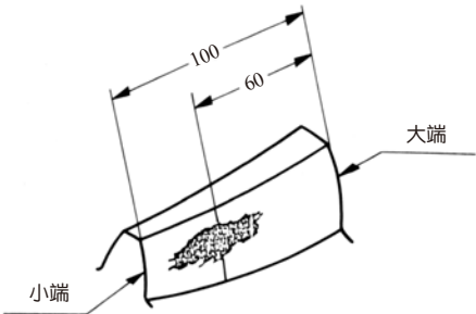
图 8.2 中央靠近小端接触
