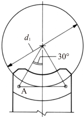
图 4.22 计算鼓形修形量的点 A
