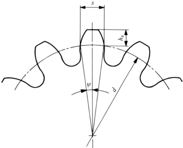
图 5.1 弦齿厚法
