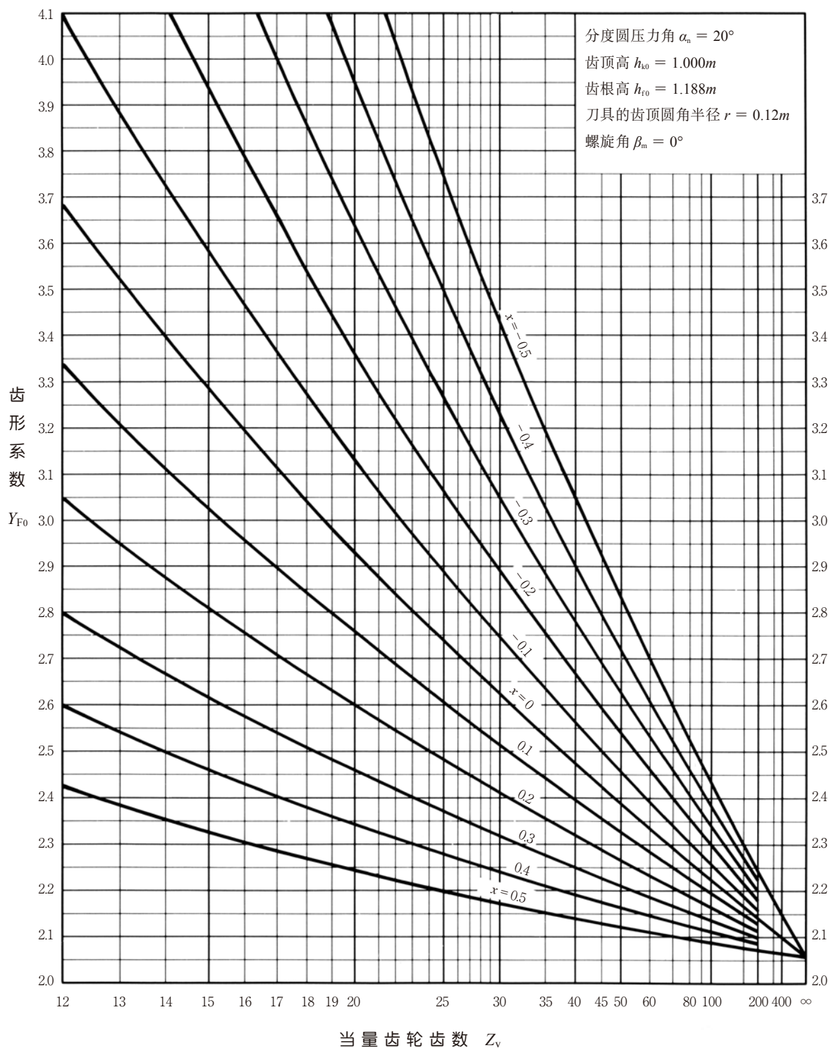
图 10.8 齿形系数 Y_{F0} (直齿锥齿轮)
