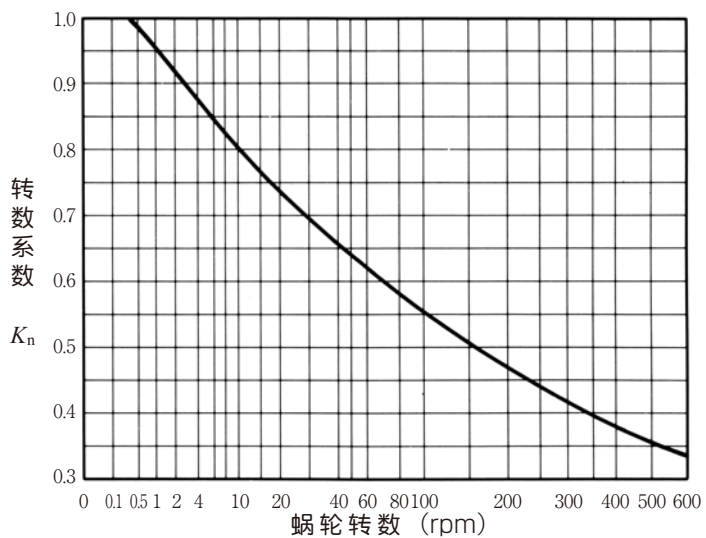
图 10.15 转数系数 K_n
