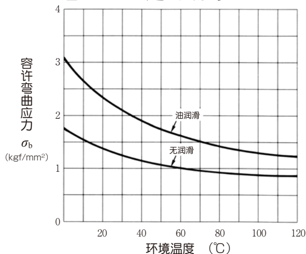
图 11.1 容许弯曲应力 \sigma_b
