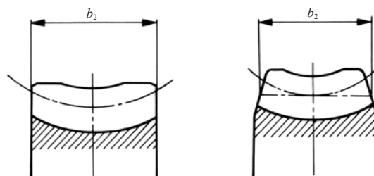
图 10.13 蜗轮的齿宽 b_2
