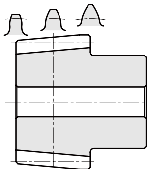
图 6.6 锥形正齿轮的齿形
