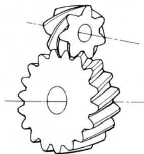
图 1.11 交错斜齿齿轮
