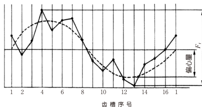
图 7.8 齿轮 (齿数为 16) 的径向跳动
