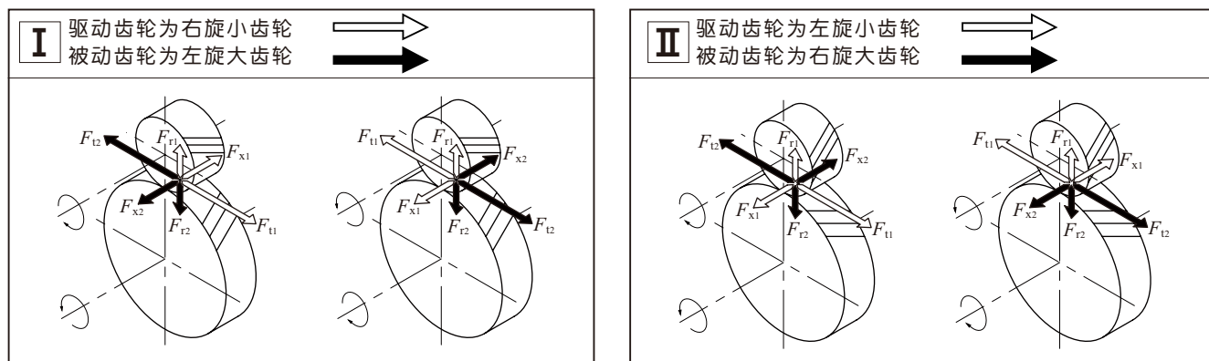
图 12.2 斜齿齿轮的旋转方向与轮齿受力
