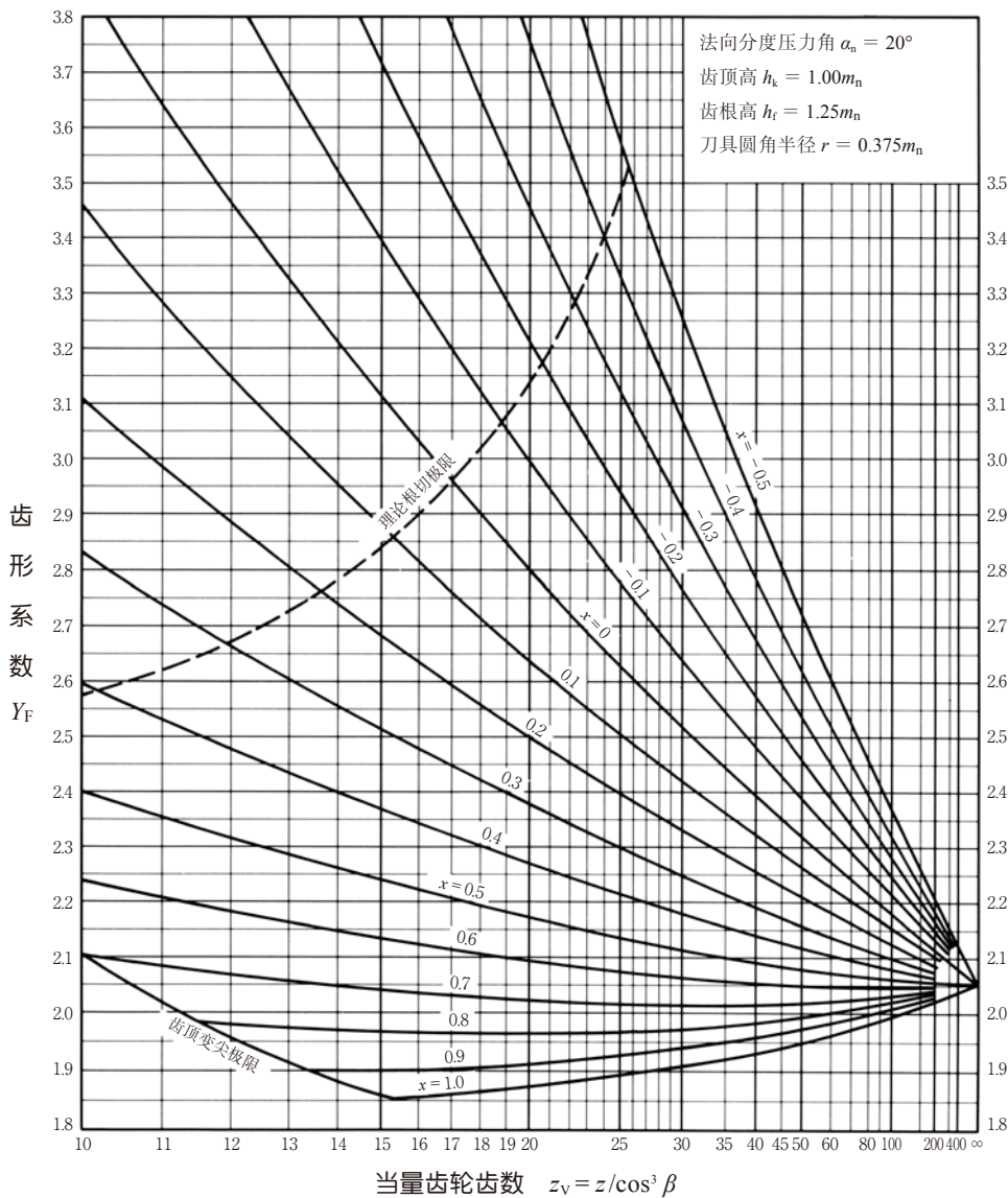
图 10.1 齿形系数图表
