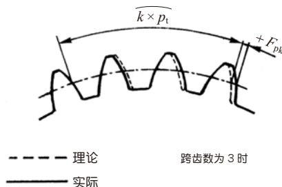
图 7.2 齿距偏差
