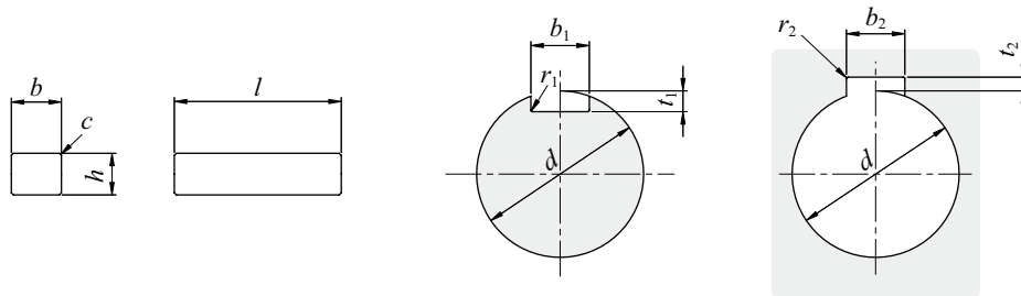
轴键槽
