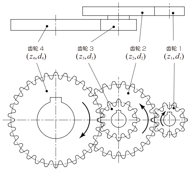
图 6.3 二级齿轮机构的侧隙
