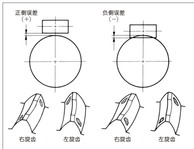
图 8.8 齿轮箱有中心距误差时的轮齿接触
