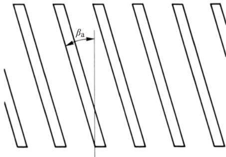
图 16.1 齿顶螺旋角的测定
