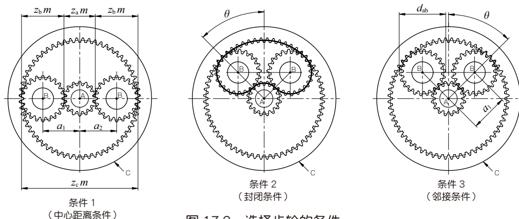
图 17.2 选择齿轮的条件
