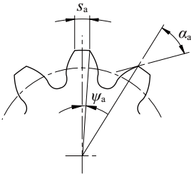
图 3.8 齿顶厚
