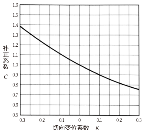
图 10.7 切向变位的修正系数 C
