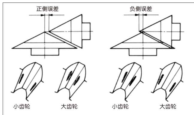
图 8.5 齿轮装配距离有误差时的轮齿接触
