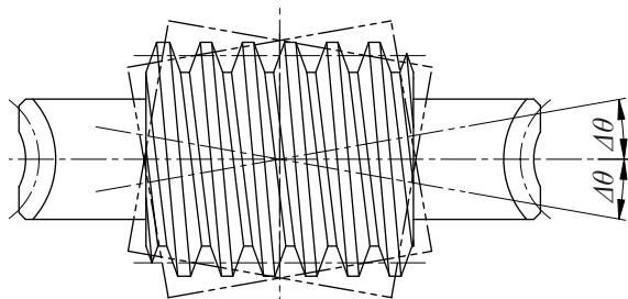
图 4.20 左右倾斜法
