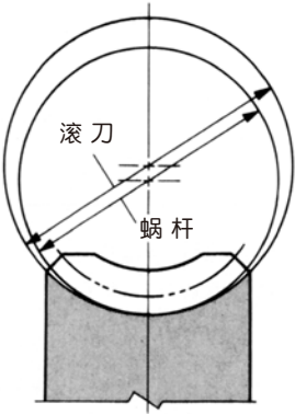
图 4.18 使用大直径滚刀的切齿方法
