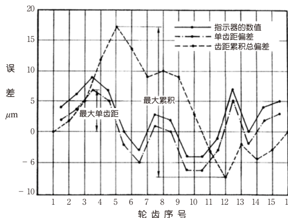
图 7.3 齿距偏差的例子
