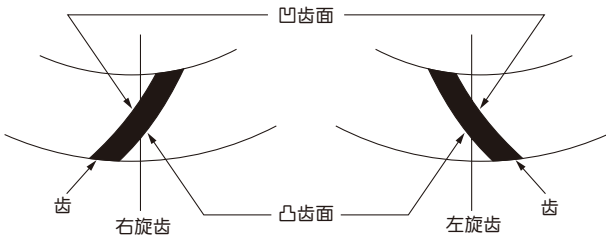
图 12.4 弧齿锥齿轮的凸齿面和凹齿面
