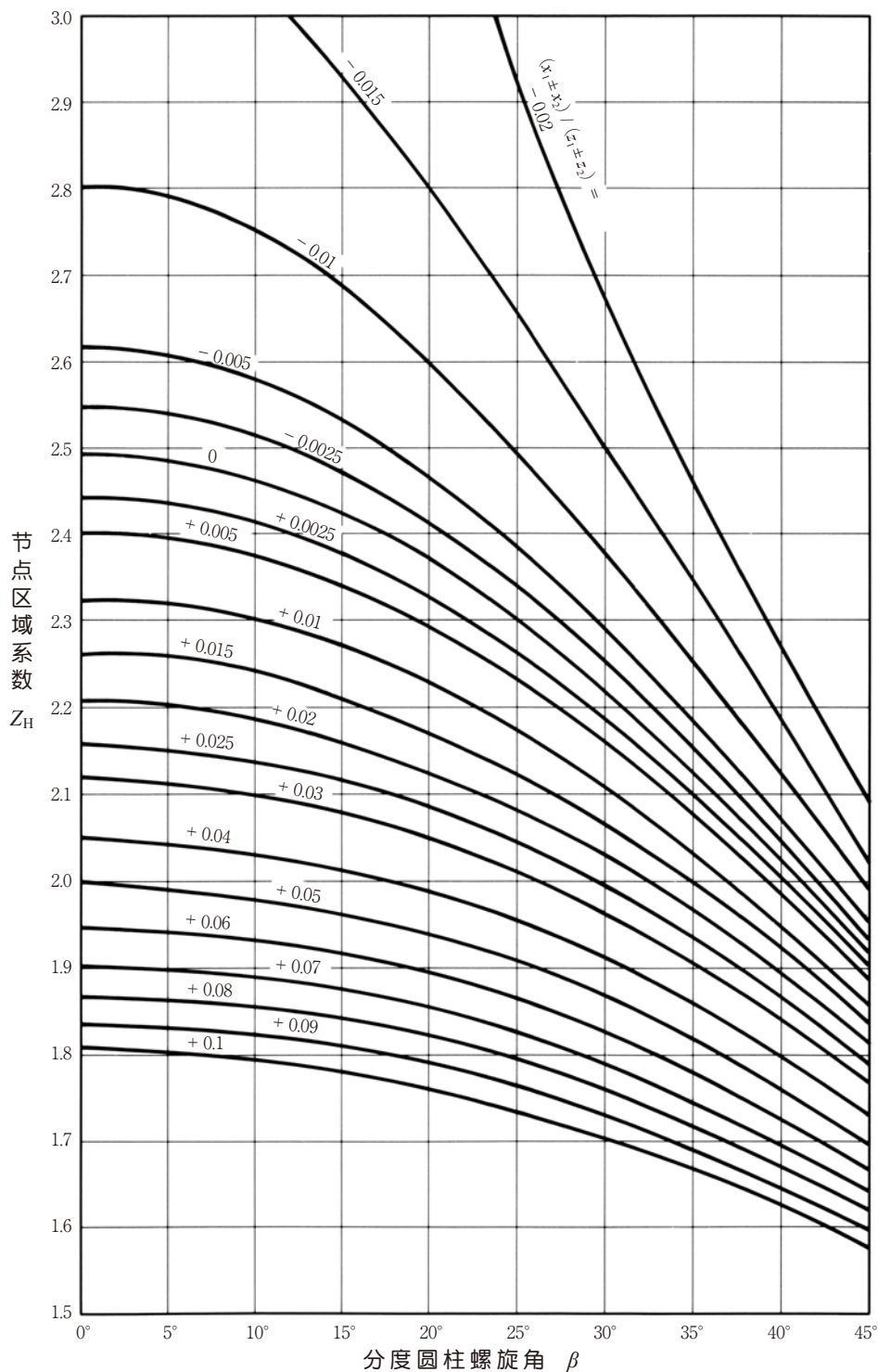
图 10.2 节点区域系数 Z_H
