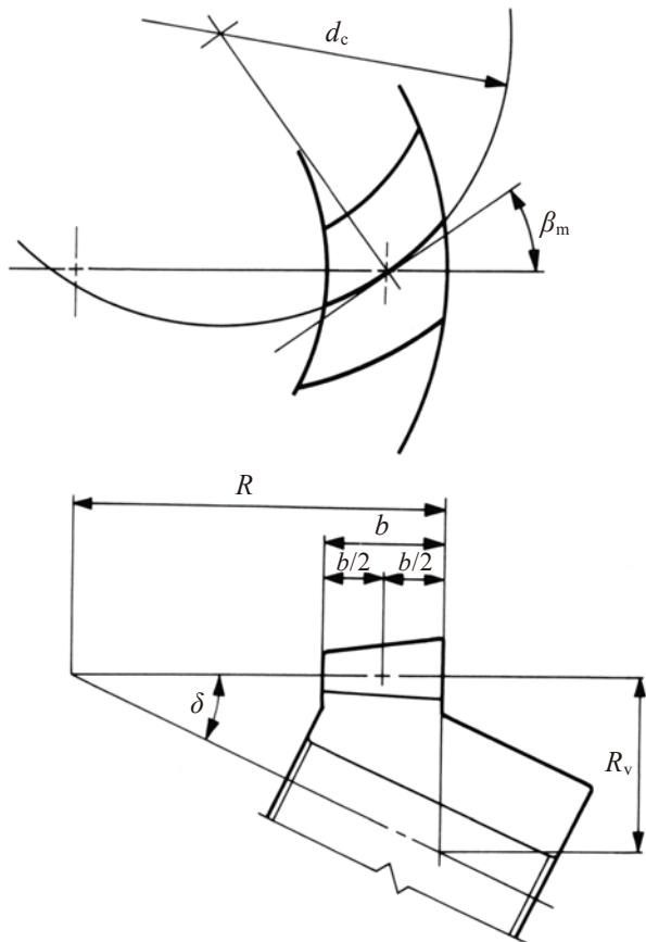
图 4.12 弧齿锥齿轮（左旋）
