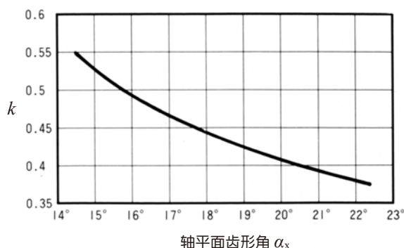
图 4.21 系数 k 值
