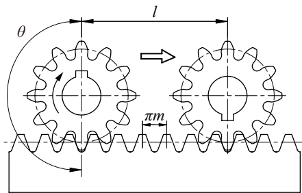
图 2.2 小齿轮和齿条
