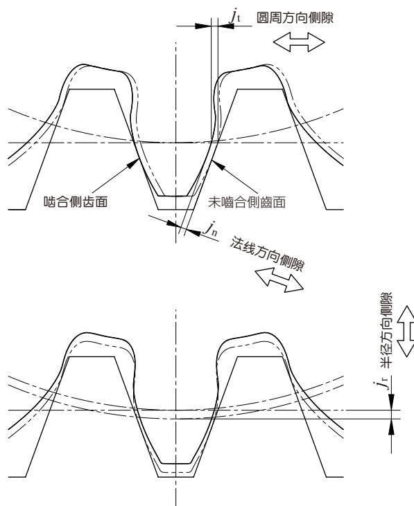
图 6.1 圆周方向 / 法线方向及半径方向的侧隙
