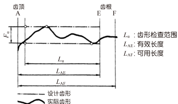
图 7.4 齿形总偏差 F_a
