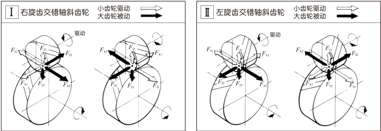
图 12.7 交错轴斜齿轮的旋转方向及轮齿受力
