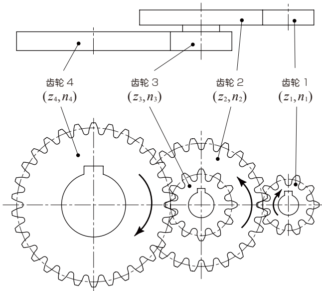
图 2.3 二级齿轮机构
