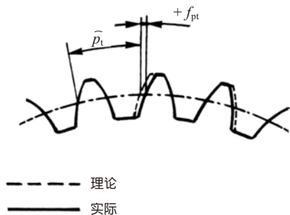
图 7.1 单齿距偏差 f_{pt}
