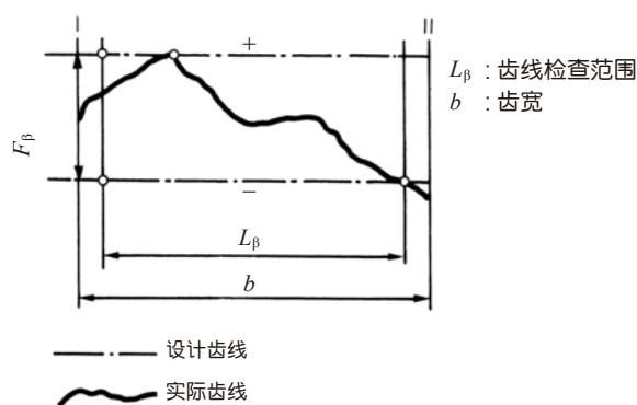
图 7.5 齿线总偏差 F_\beta
