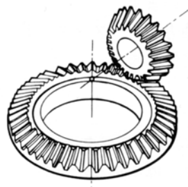
图 1.9 零度锥齿轮
