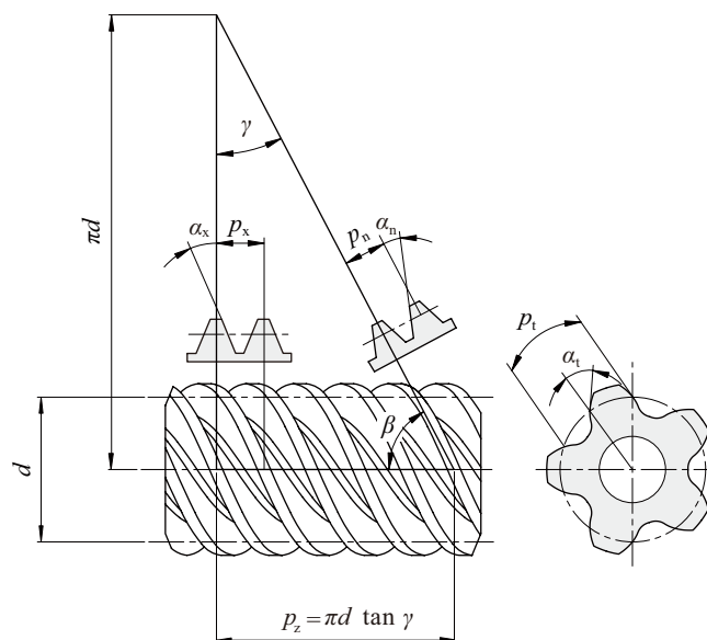
图 4.16 圆柱蜗杆（右螺旋）
