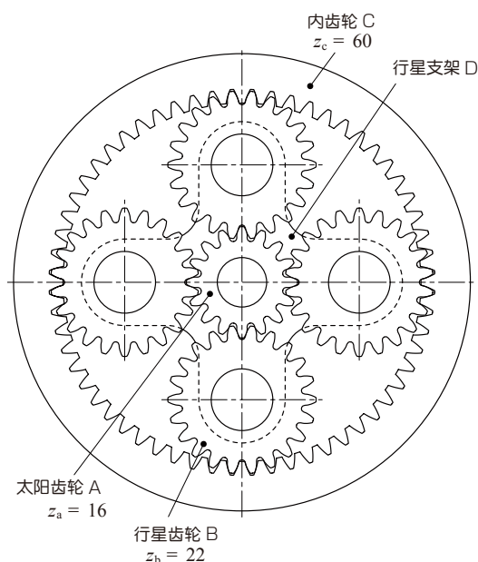
图 17.1 行星齿轮机构的构造
