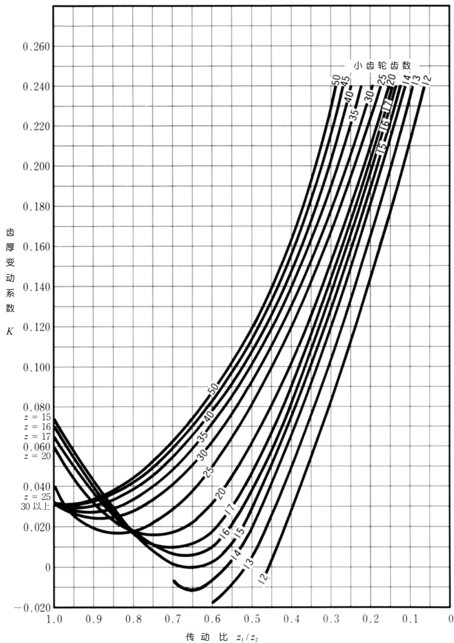
图 5.3 格里森弧齿锥齿轮的齿厚变动系数 K 线图
