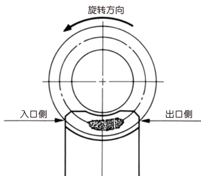
图 8.6 理想的轮齿接触
